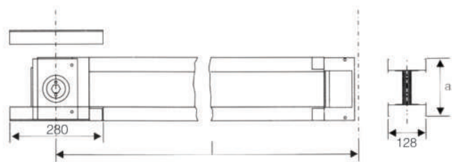
单排系统
