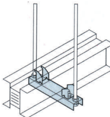
水平侧装使用
